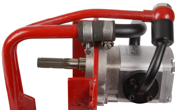
Ersättningsutförande med ombyggnadssats monterad, sedd från höger sida.
