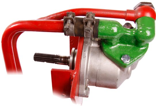
Ursprungligt utförande av hydraulpumpens montering, sedd från höger sida.
